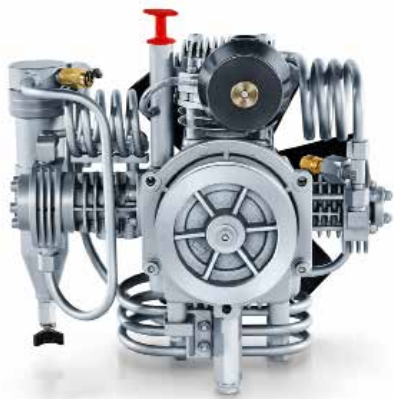
PE 100 Compressor Block
